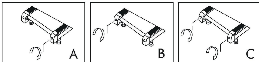
Рисунок 17 — Центровка бегового полотна
