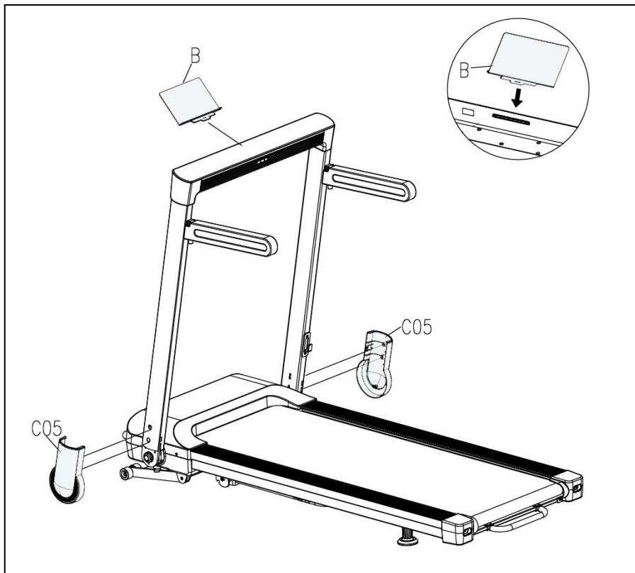
Рисунок 5 — Установка подставки для планшета и боковых накладок
