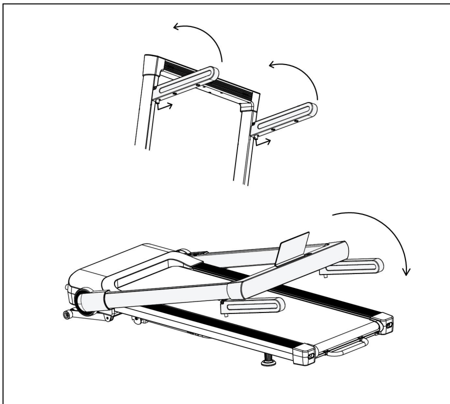
Рисунок 7 — Схема складывания стоек консоли
