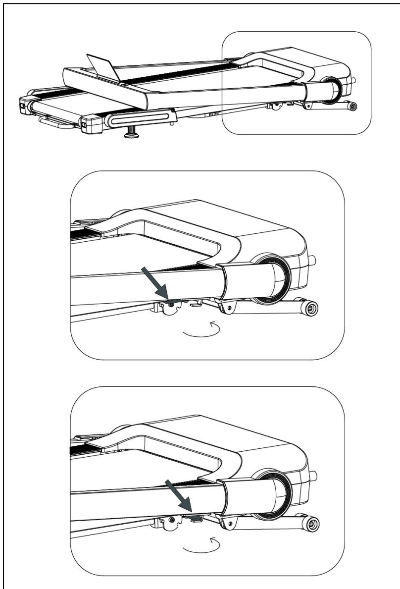
Рисунок 8 — Фиксация стоек консоли на нижней раме беговой дорожки
