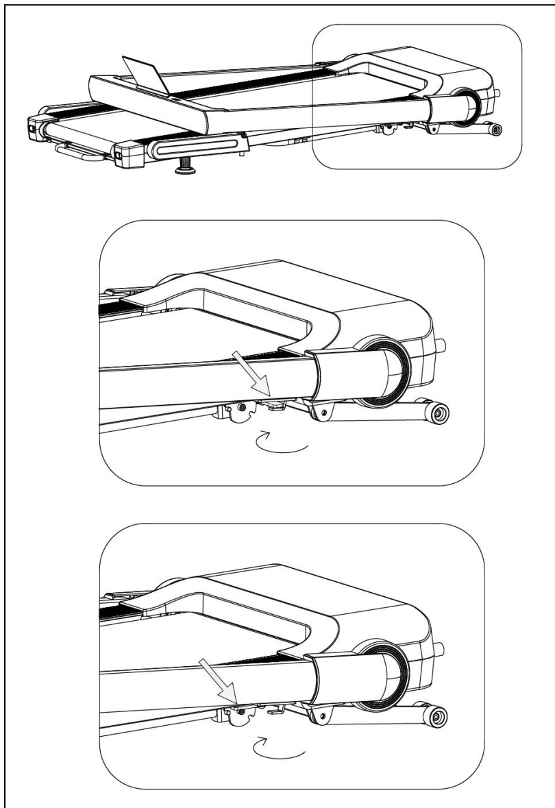
Рисунок 13 — Схема извлечения пластины из крючка
