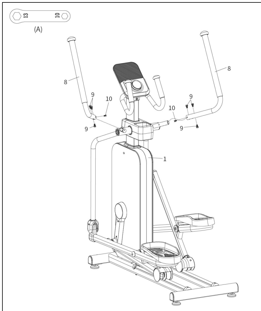
Рисунок 7 — Установка поручней
