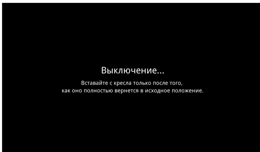
Рисунок 40 — Экран выключения
