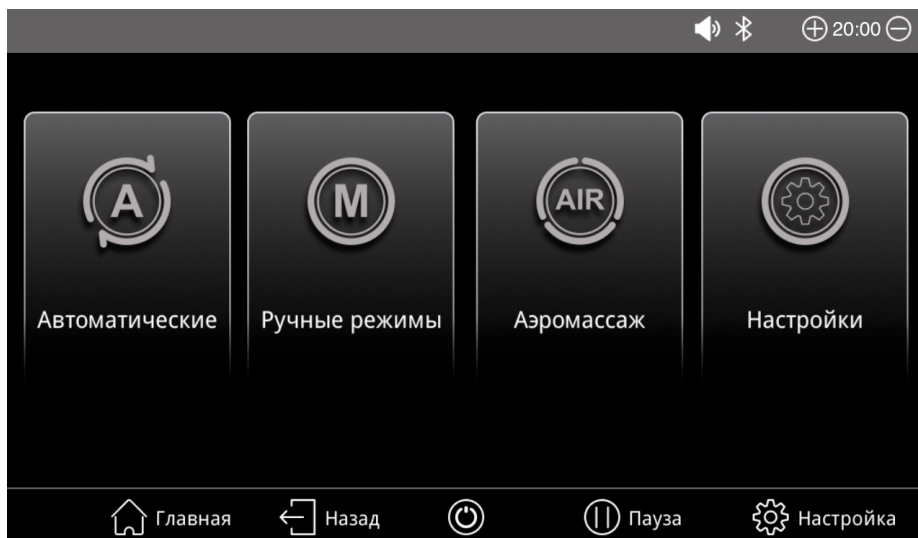
Рисунок 29 — Главный экран
