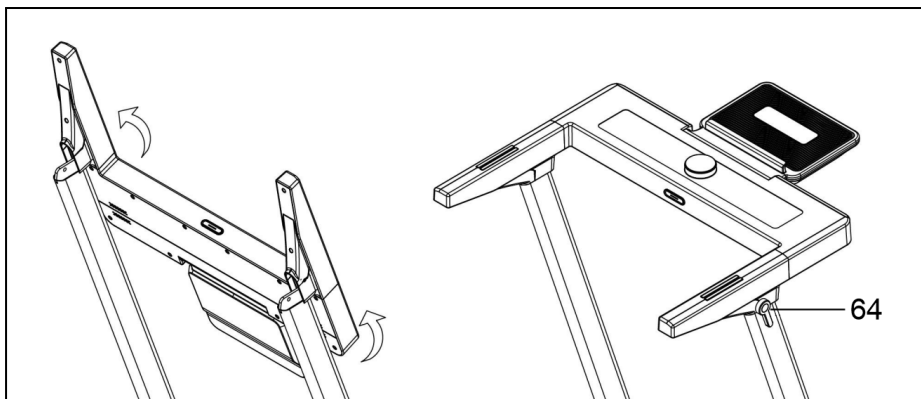
Рисунок 3 — Установка и фиксация консоли
