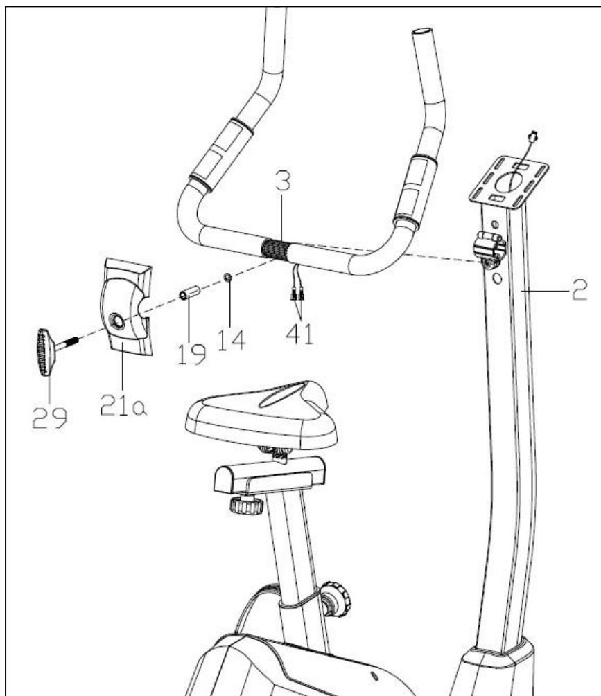
Рисунок 6 — Установка поручней
