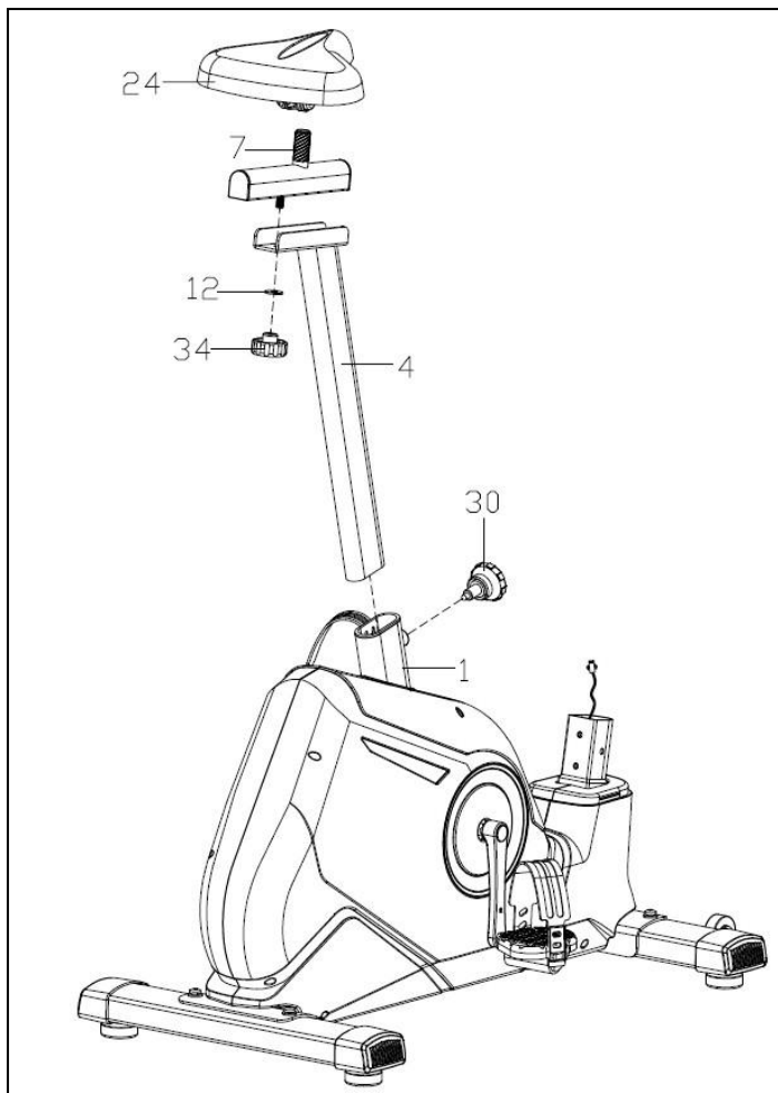
Рисунок 4 — Установка седла
