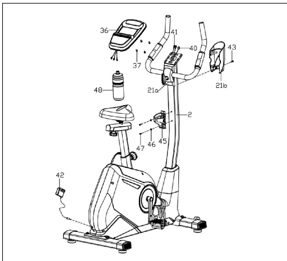
Рисунок 7 — Установка консоли и держателя для бутылки
