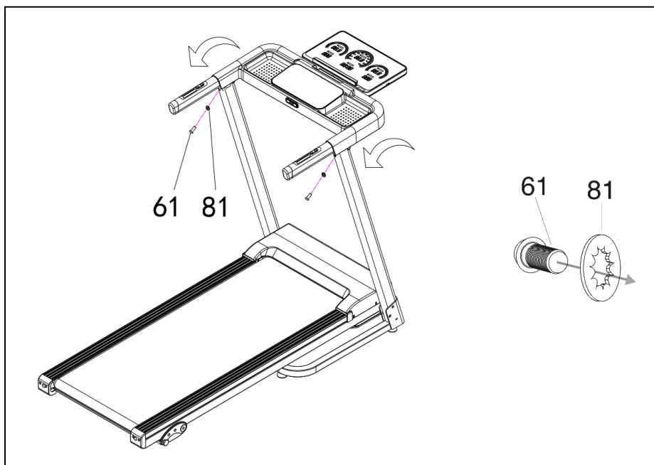
Рисунок 4 — Установка консоли беговой дорожки
