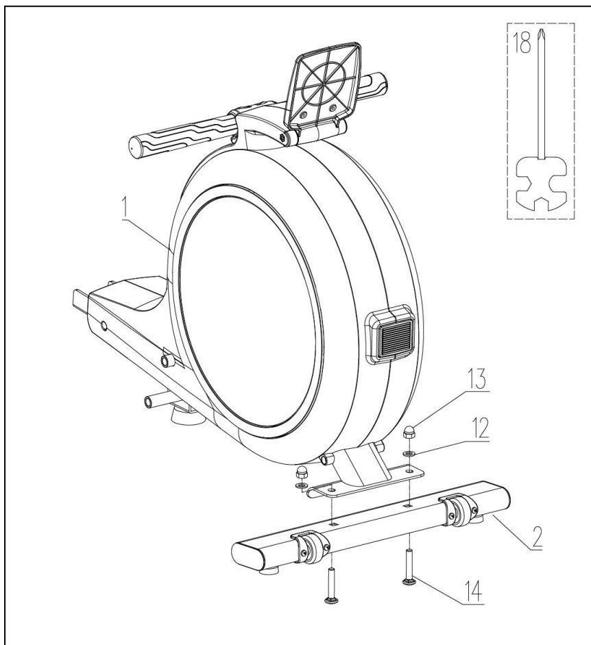
Рисунок 2 — Установка передней опоры
