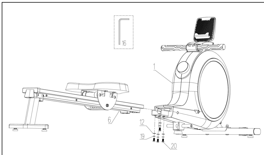
Рисунок 4 — Сборка основной рамы
