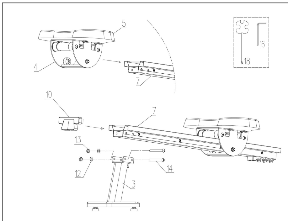
Рисунок 3 — Установка сиденья и задней опоры
