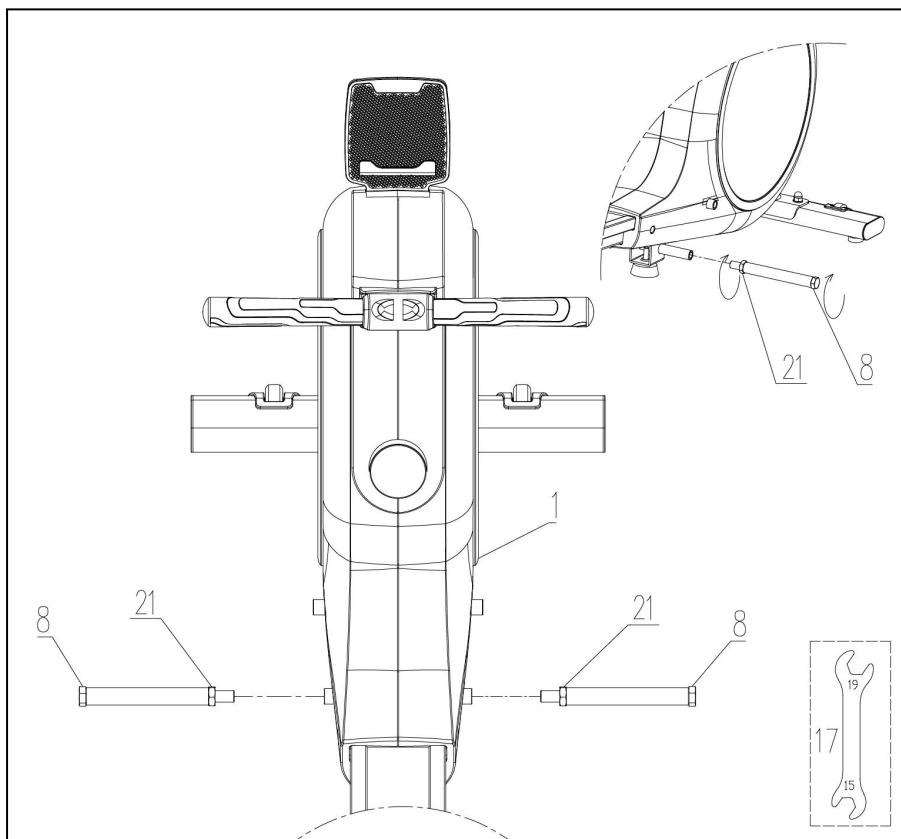
Рисунок 5 — Установка pedalных стоек
