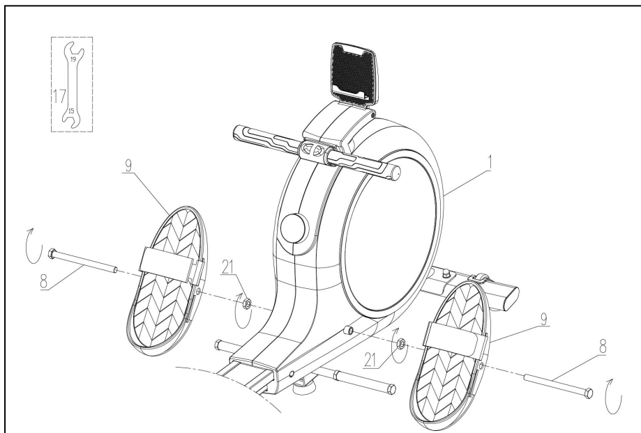
Рисунок 6 — Установка педалей
