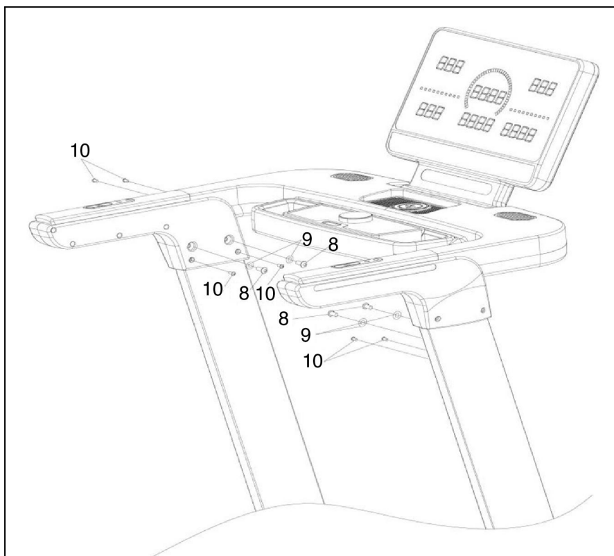
Рисунок 4 — Установка консоли
