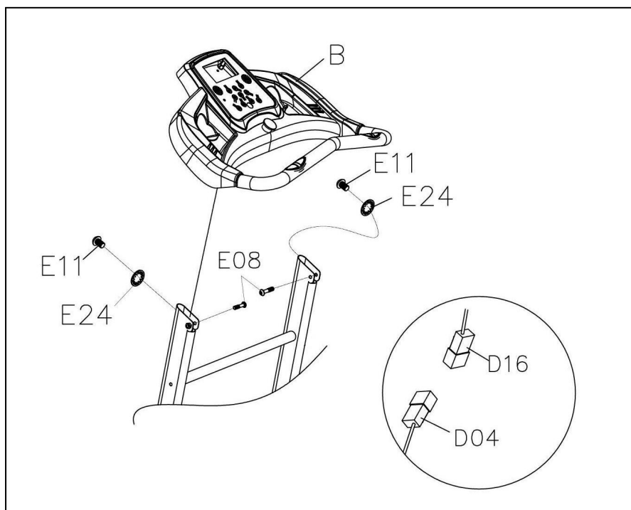
Рисунок 4 — Установка консоли
