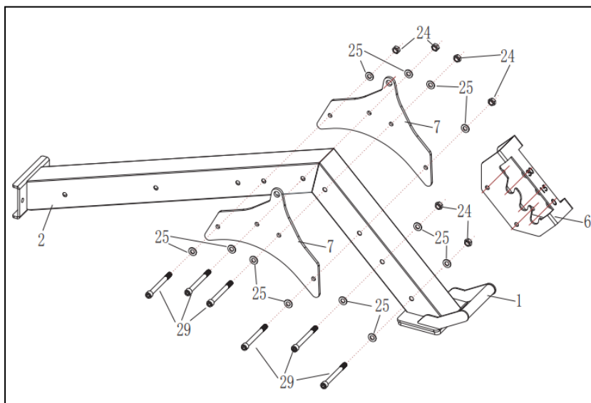
Рисунок 1 — Установка опорного подрамника и ограничителя положения сиденья
