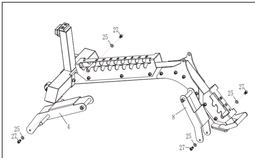
Рисунок 5 — Установка рамы регулировки положения спинки и рамы регулировки положения сиденья
