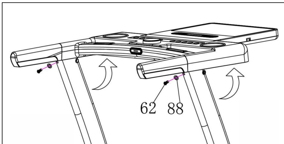
Рисунок 3 — Установка консоли
