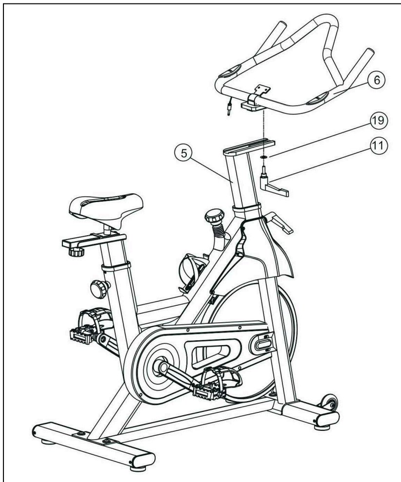
Рисунок 6 — Установка руля
