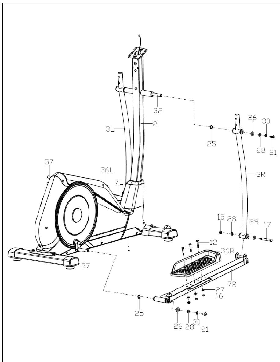
Рисунок 4 — Установка педалей
