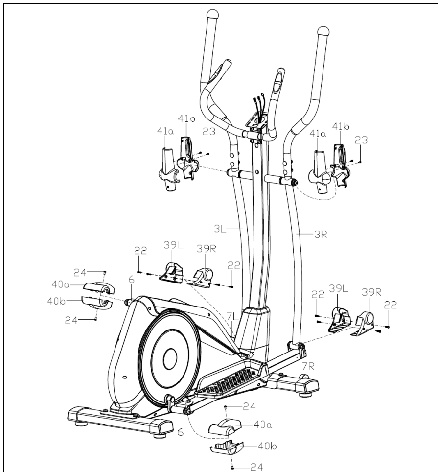
Рисунок 6 — Крепление кожуhов
