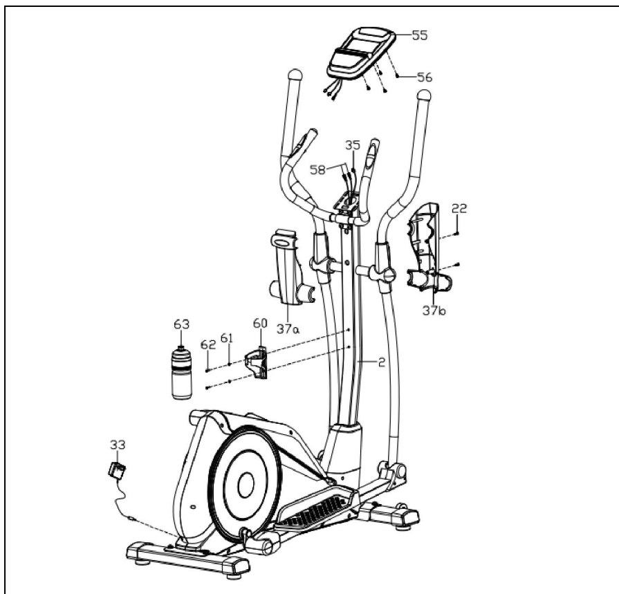
Рисунок 7 — Установка консоли и держателя для бутылки
