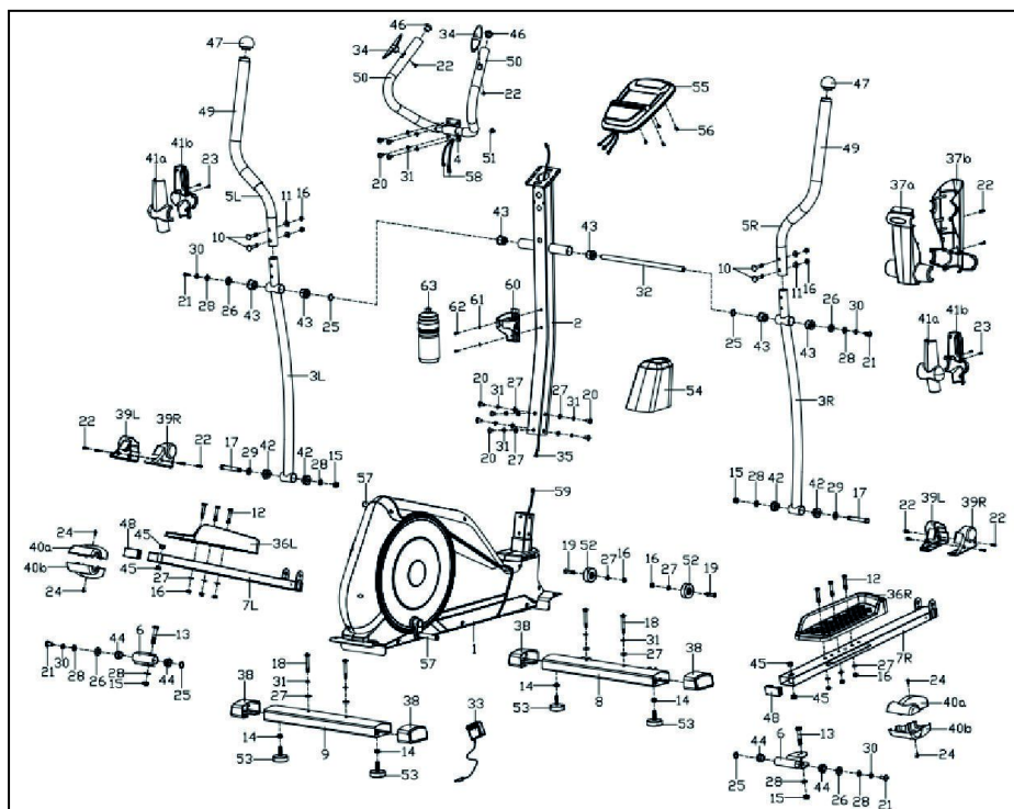
Рисунок 1 — Схема тренажера в разобранном виде
