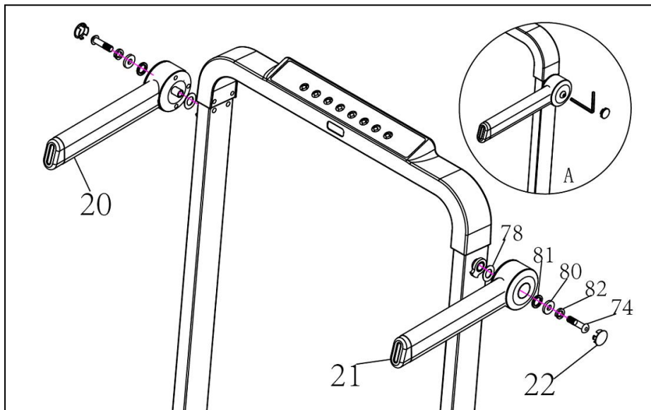
Рисунок 4 — Фиксация поручней
